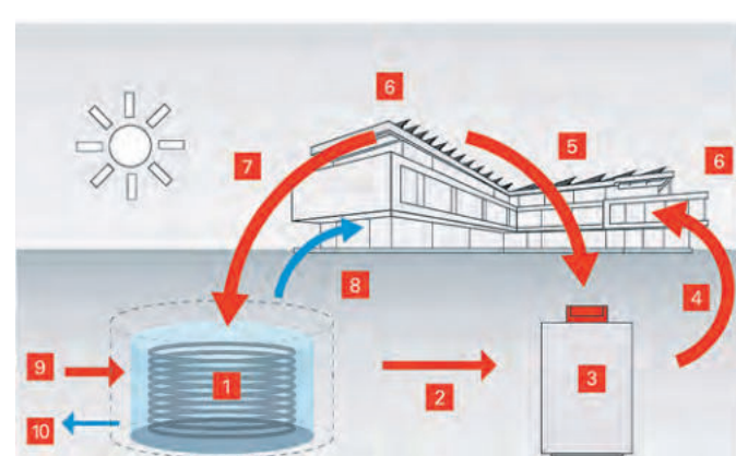
Schematische Darstellung des Eisspeichers.
